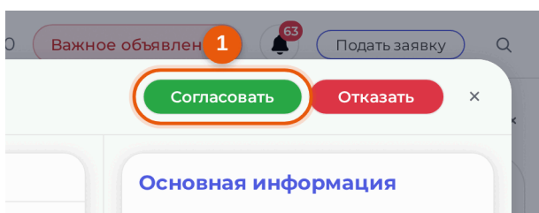
Рисунок 7.1 — Кнопки решения
